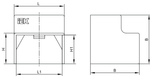
Рисунок 2 – Угол Т-образный КМТ / Figure 2 – T-bend KMT / 2-сурет – Т-тәрізді бұрыш КМТ
