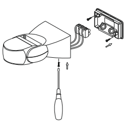
Рисунок 16 – Монтаж ДД 013
