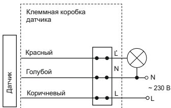
Рисунок 22 – Схема подключения датчиков типов: ДД 013, ДД 016
