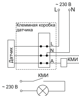
Рисунок 29 – Схема подключения датчика с контактором КМИ
