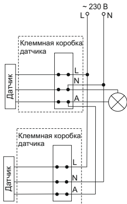
Рисунок 27 – Схема параллельного подключения датчиков
