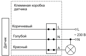
Рисунок 23 – Схема подключения датчиков типов: ДД 015, ДД 022, ДД 023
