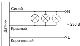
Рисунок 26 – Схема подключения датчиков типов: ДД 046
