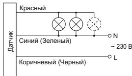
Рисунок 24 – Схема подключения датчиков типов: ДД 041
